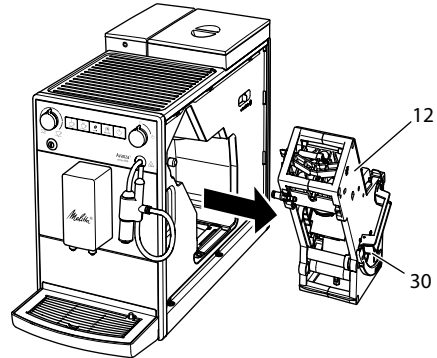
Fig. 16: Afmontering af brygheden
