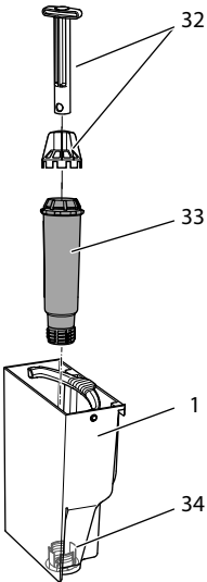
Bild 19: Skruva fast eller lossa vattenfiltret
