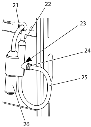
Kuva 4: Cappuccinatore
