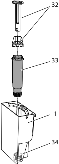
Kuva 19: Vesisuodattimen ruuvaaminen paikalleen tai irti
