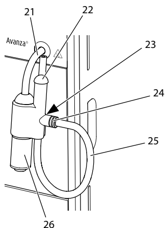
Bild 4: Cappuccinatore
