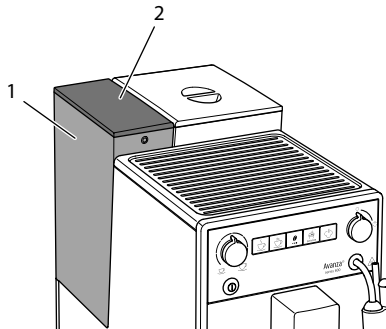
Kuva 8: Vesisäiliön poistaminen
