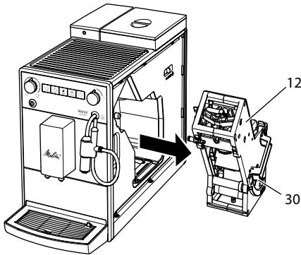
Abb. 16: Brühgruppe ausbauen
